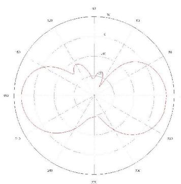
E-Plane
